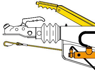
Auflaufeinrichtung mit ölhydraulischer Ansteuerung
